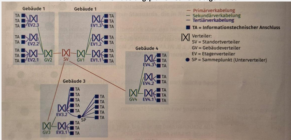
Schematischer Verkabelungsplan eines Betriebsgeländes
